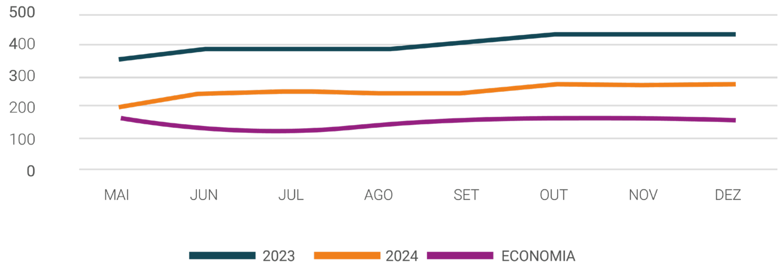
DEMONSTRAÇÃO DA REDUÇÃO DO CUSTO DE ENERGIA ELÉTRICA – MAIO A DEZ DE 2024
